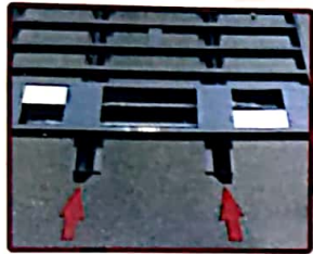
Rieles formados para guiar la carrocería, aseguran la correcta alineación con el sistema de levantamiento del chasis.
