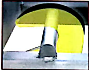
Barras en acero que aseguran la carrocería al chasis con bloqueo para seguridad añadida.
